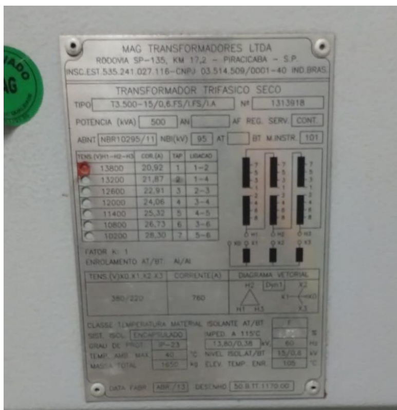
Placa do transformador
